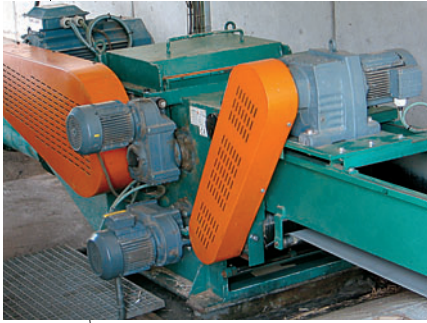
Astilladora de tambor con alimentación mediante banda transportadora. Drum chipper with belt conveyor infeed.
