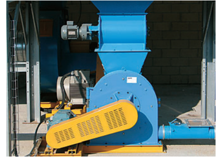
Refinador con rotor de martillos oscilantes. Refiner with swinging hammers rotor.
