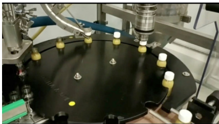
* Conjunto de alimentación de tapón y roscado automático
